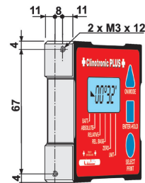
Linke Abbildung: Clinotronic PLUS mit Magneteinsätzen links und unten z.B. 015-PLUS-FG45
