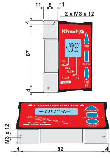
Linke Abbildung: CLINOTRONIC PLUS mit Magneteinsätzen links und unten / z.B. 015-PLUS-FG45
